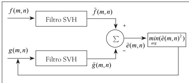
Figura 20. Esquema genérico de DBS
